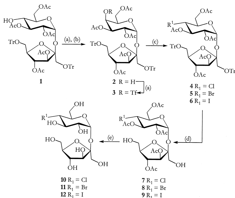
Scheme 1. (a) Tf 2 O, pyridine/CH 2 Cl 2 ; (b) NaNA 2 , DMF, rt, (c) 4 : LiCl, acetone, rt, 5 : LiBr, acetone, rt; 6 : KI, acetone, rt; (d) AcOH-CH 2 Cl 2 (1:1), concd HCl, 0 °C; (e) NaOMe, MeOH, rt.
